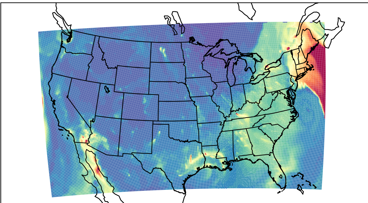
WRF 2023-12-18_14:00:00
