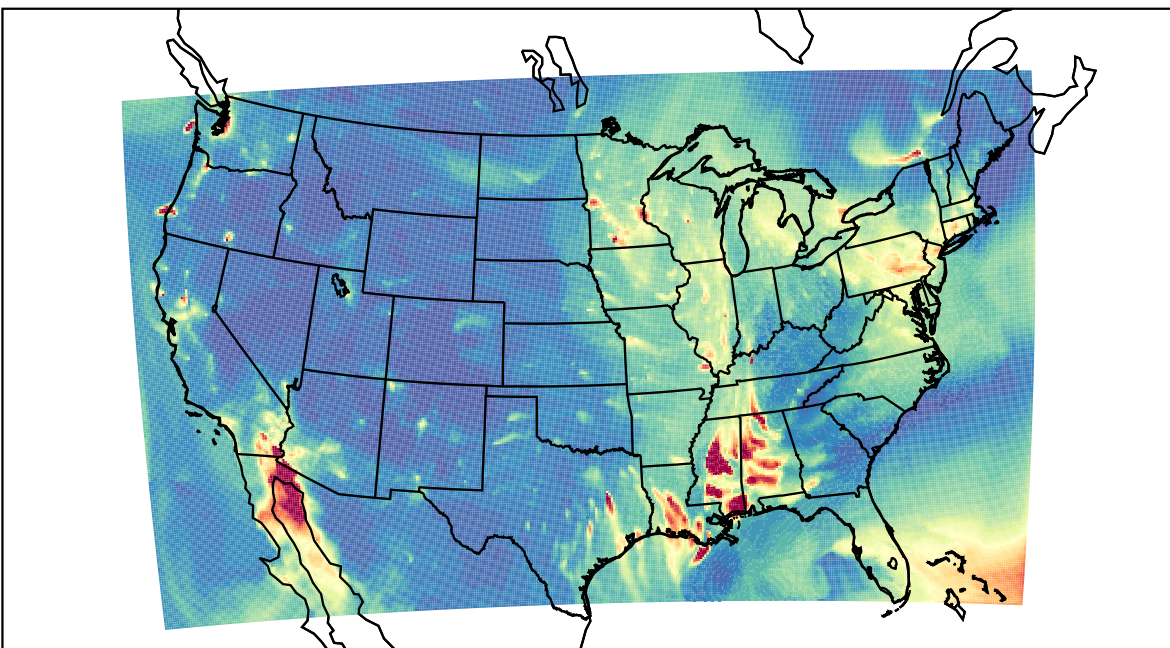
WRF 2023-12-17_04:00:00
