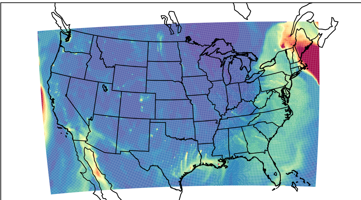
WRF 2023-12-18_20:00:00
