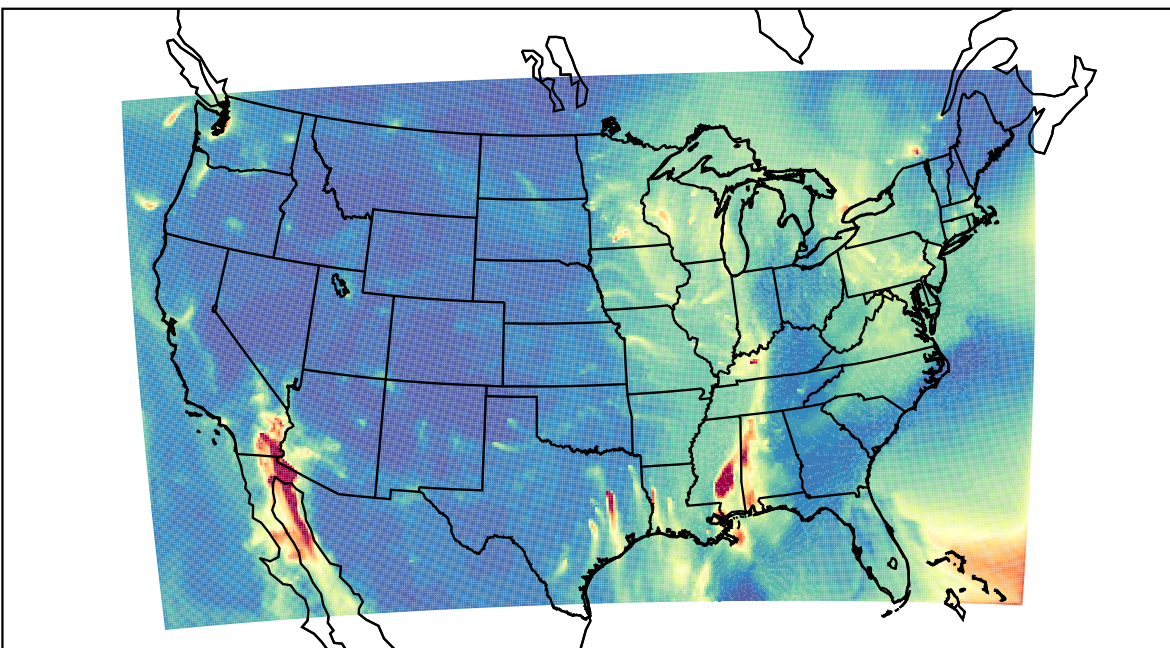
WRF 2023-12-17_10:00:00
