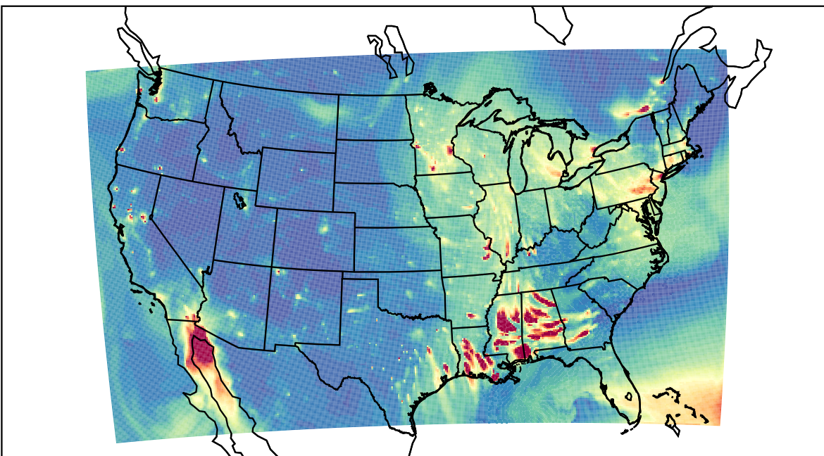
WRF 2023-12-17_01:00:00
