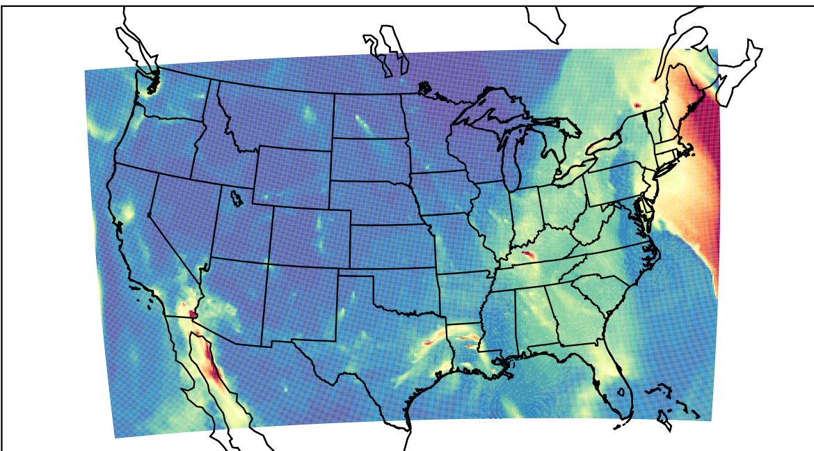
WRF 2023-12-18_10:00:00
