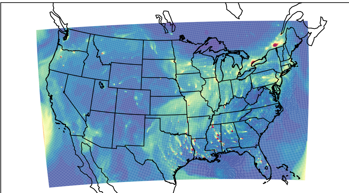
WRF 2023-12-20_22:00:00
