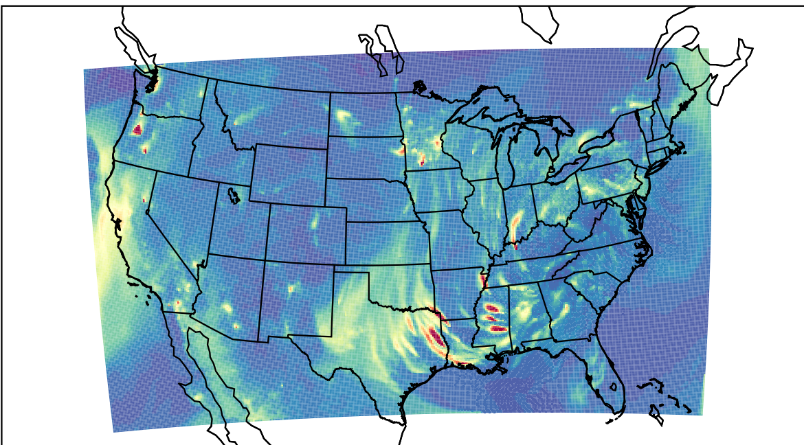
WRF 2023-12-20_04:00:00
