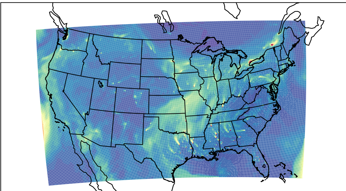
WRF 2023-12-20_19:00:00
