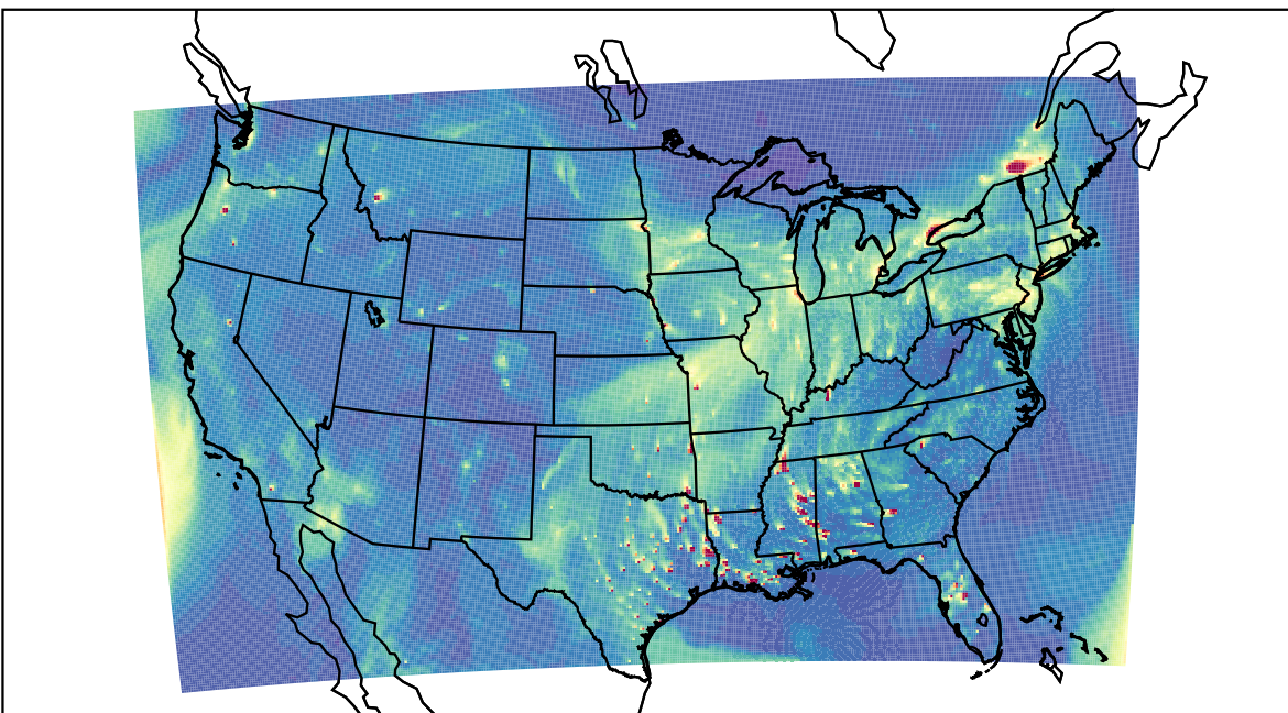
WRF 2023-12-20_23:00:00
