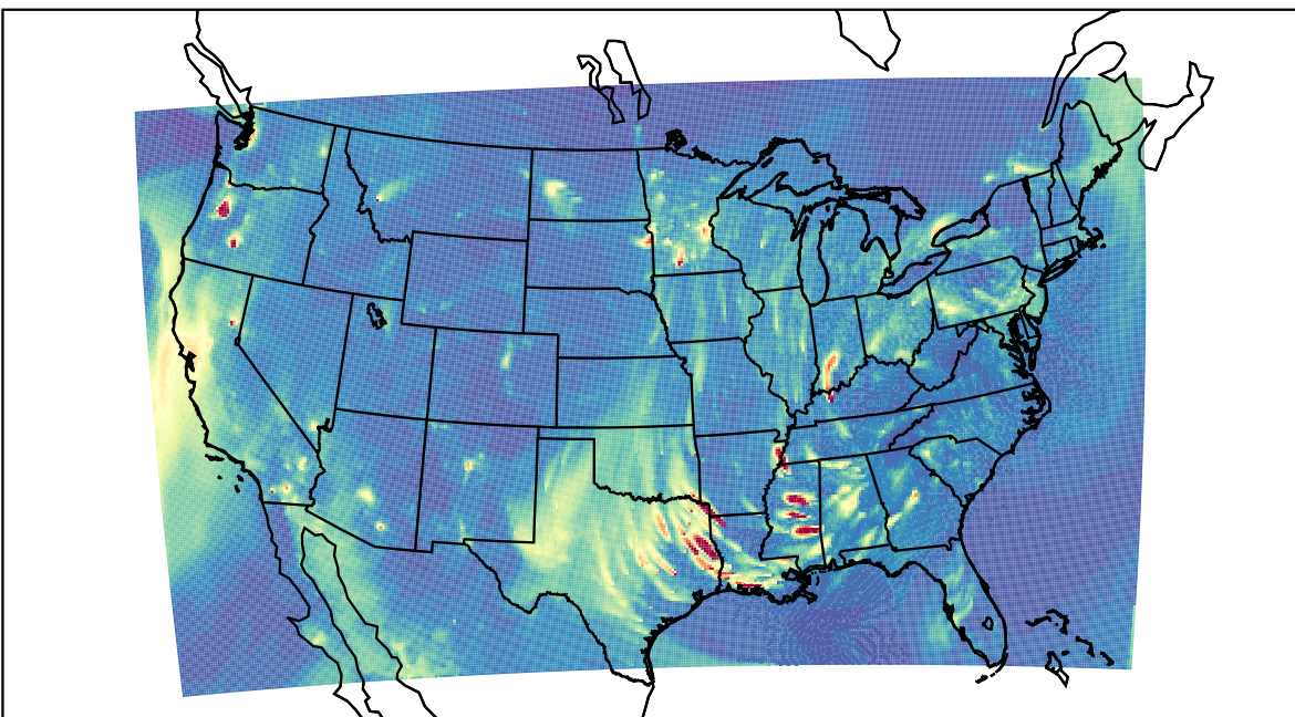
WRF 2023-12-20_03:00:00
