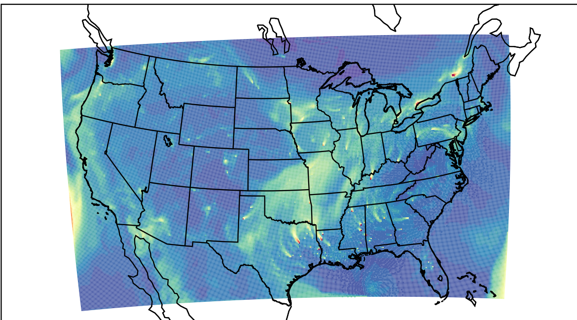
WRF 2023-12-20_18:00:00
