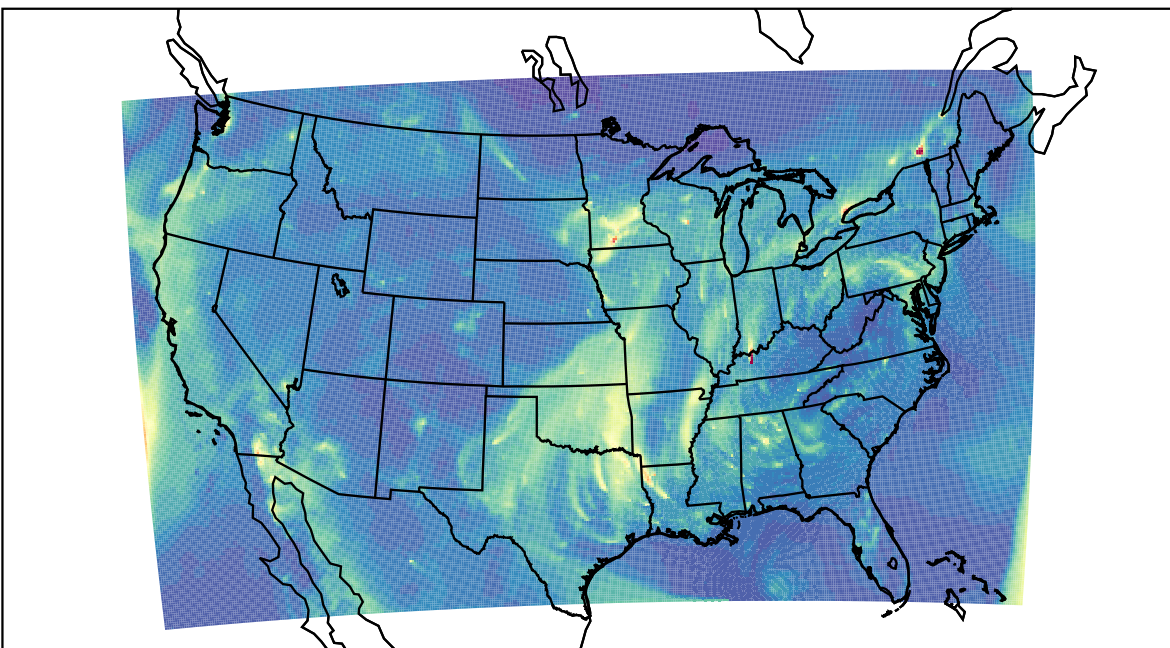
WRF 2023-12-20_14:00:00
