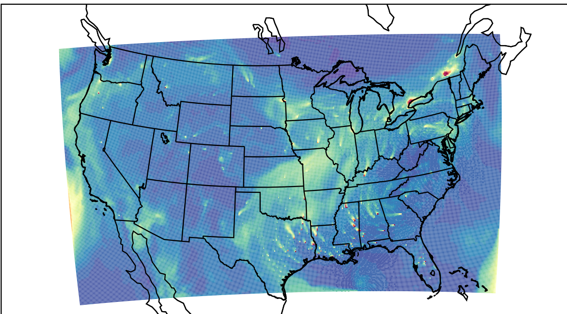
WRF 2023-12-20_20:00:00
