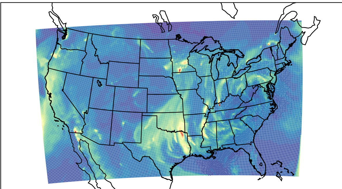
WRF 2023-12-20_10:00:00
