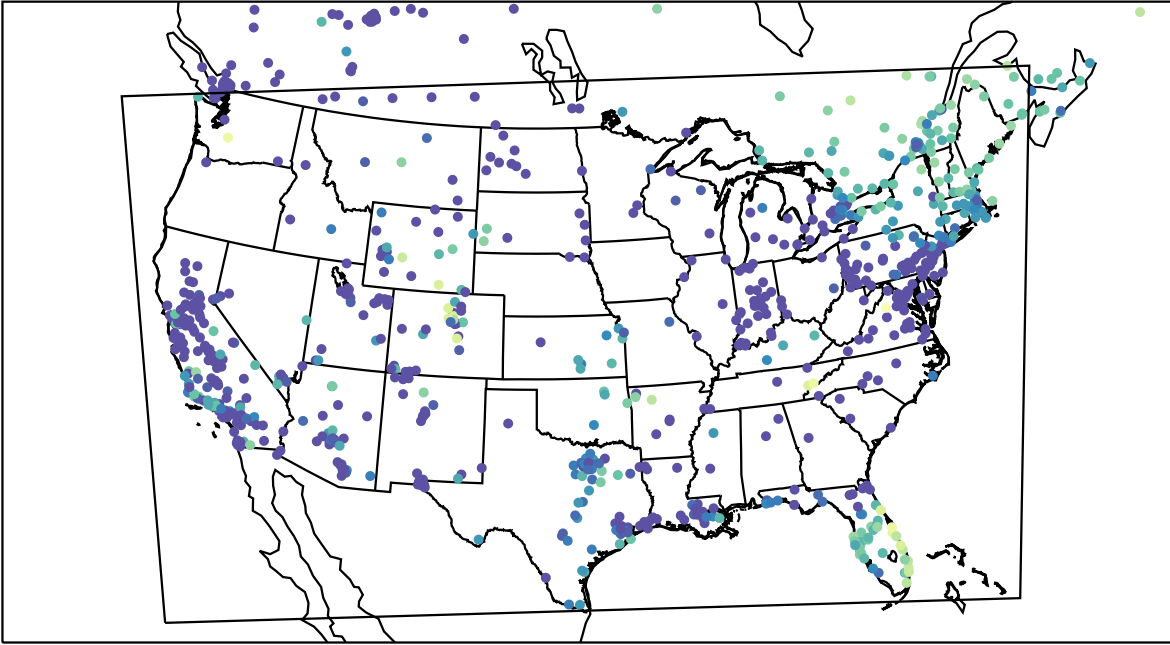
AirNOW (2023-12-21_13:00:00)
