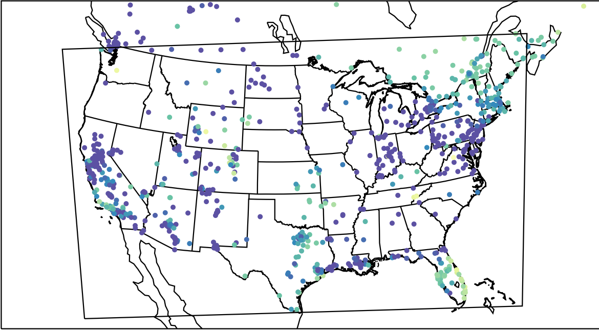
AirNOW (2023-12-21_10:00:00)
