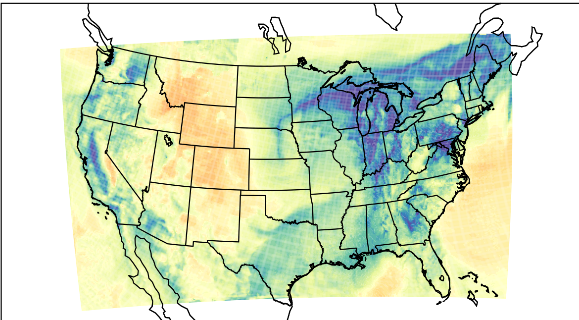
WRF (2023-12-26_18:00:00)
