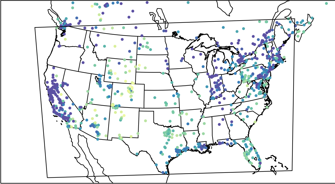
AirNOW (2023-12-26_18:00:00)
