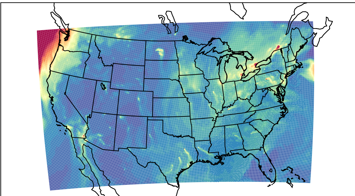
WRF 2023-12-28_18:00:00
