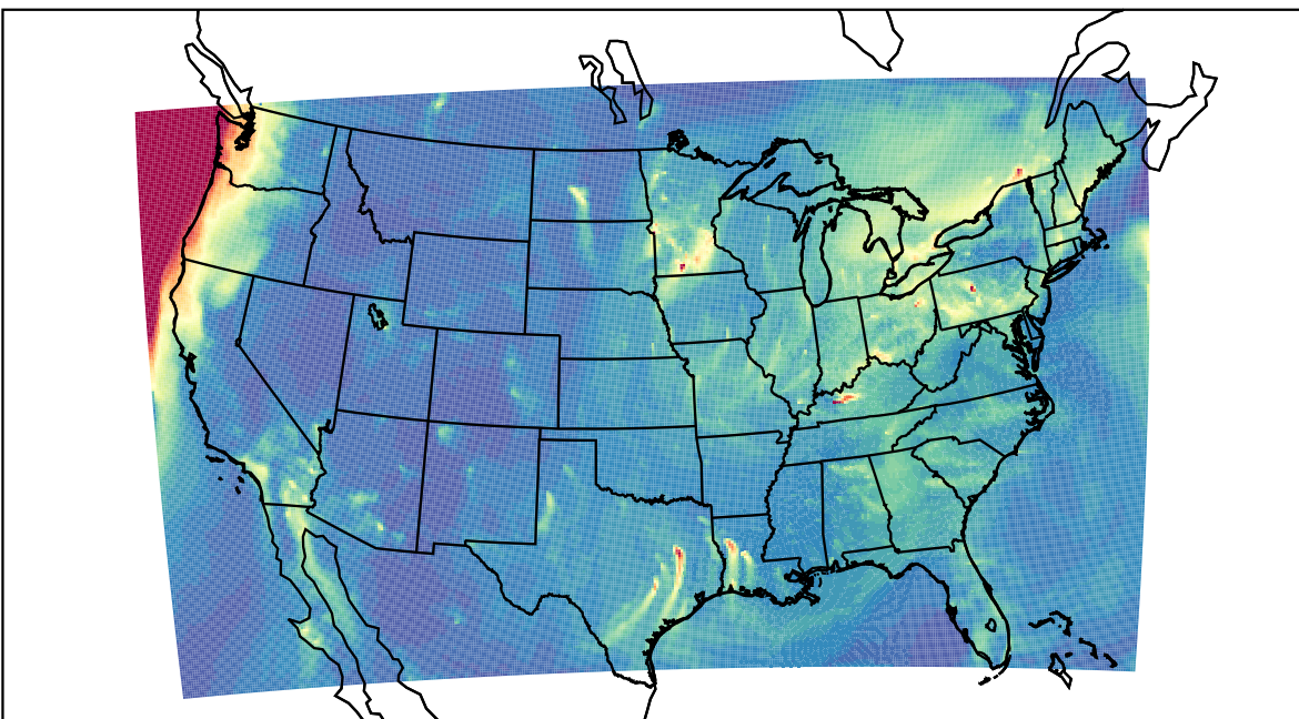
WRF 2023-12-28_10:00:00
