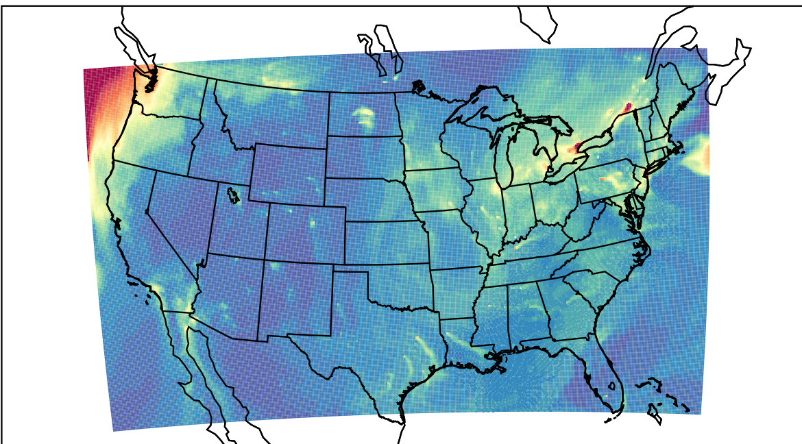
WRF 2023-12-28_20:00:00
