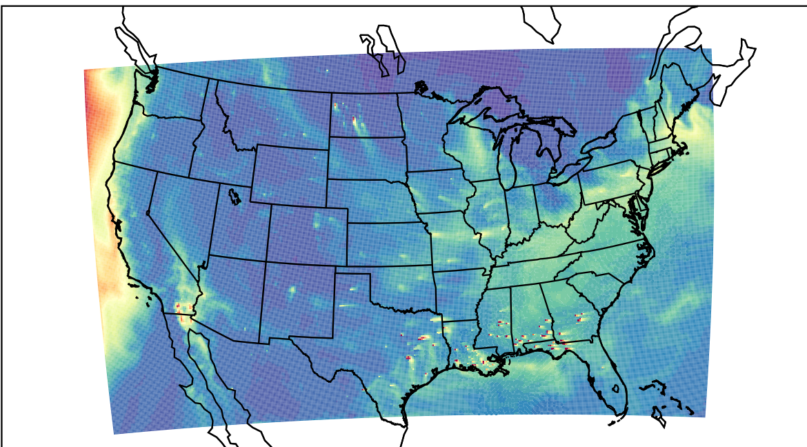
WRF 2023-12-30_18:00:00
