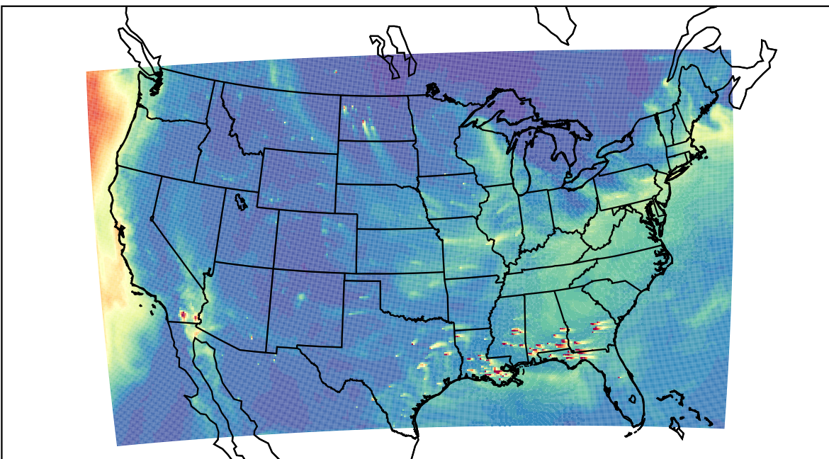
WRF 2023-12-30_20:00:00
