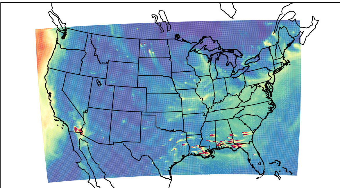
WRF 2023-12-30_22:00:00
