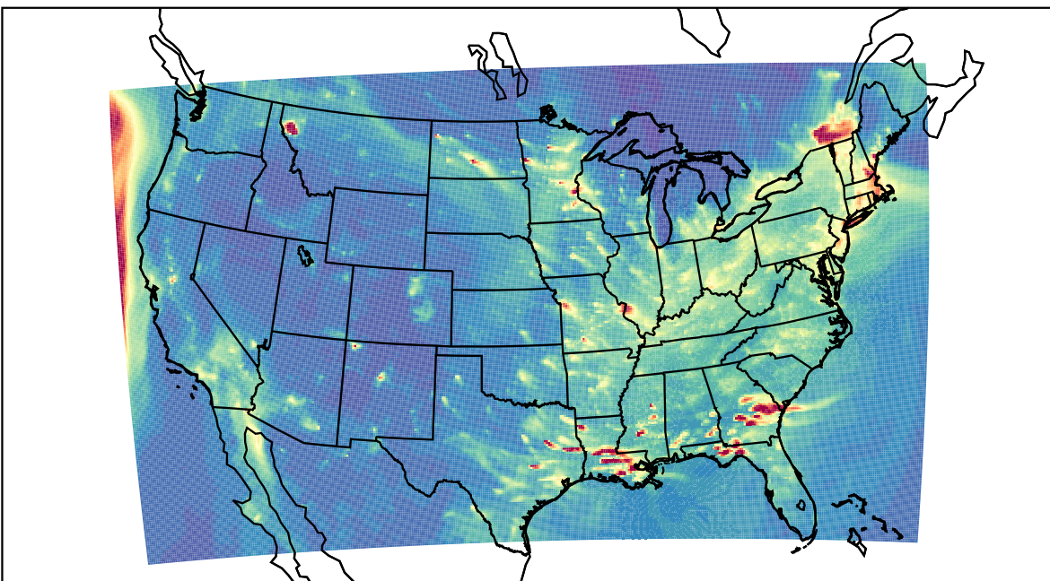
WRF 2023-12-30_03:00:00
