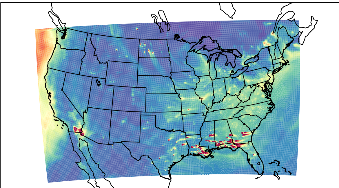
WRF 2023-12-30_23:00:00
