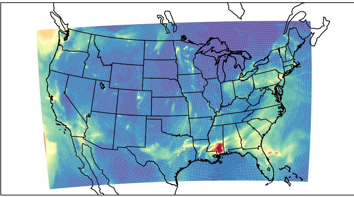
WRF 2024-01-01_09:00:00
