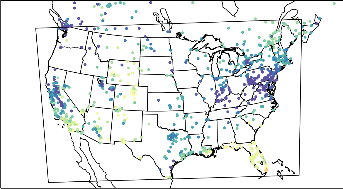
AirNOW (2024-01-01_20:00:00)
