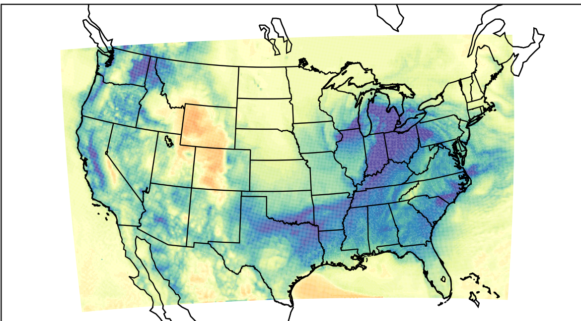
WRF (2023-12-31_16:00:00)
