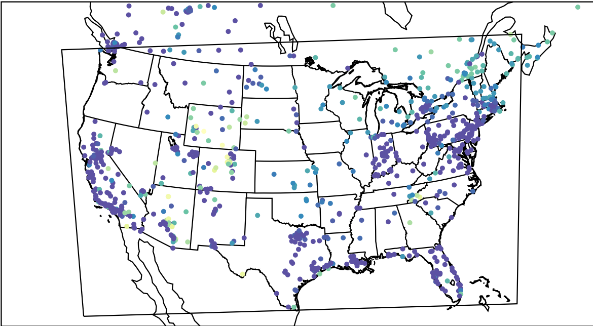
AirNOW (2024-01-01_11:00:00)
