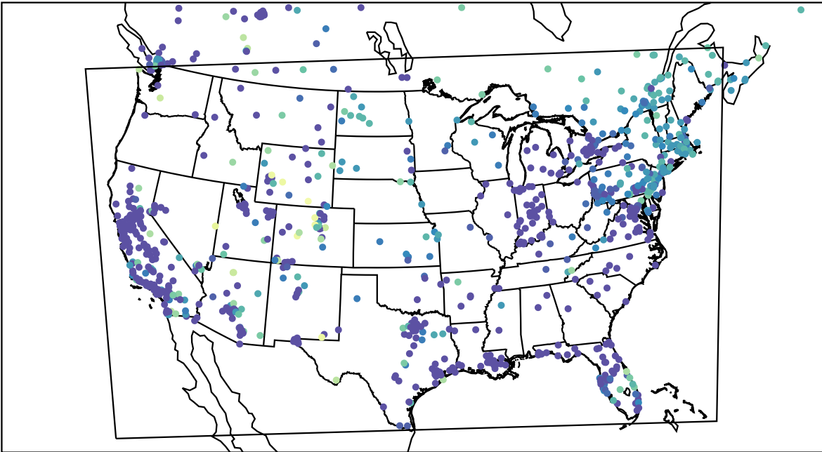
AirNOW (2023-12-31_13:00:00)
