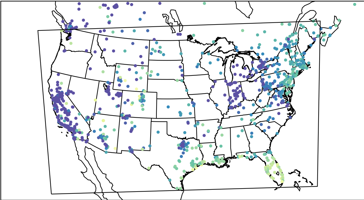
AirNOW (2023-12-31_16:00:00)
