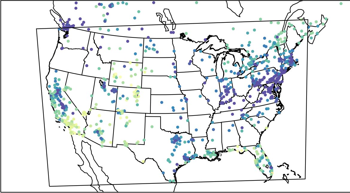
AirNOW (2024-01-01_23:00:00)
