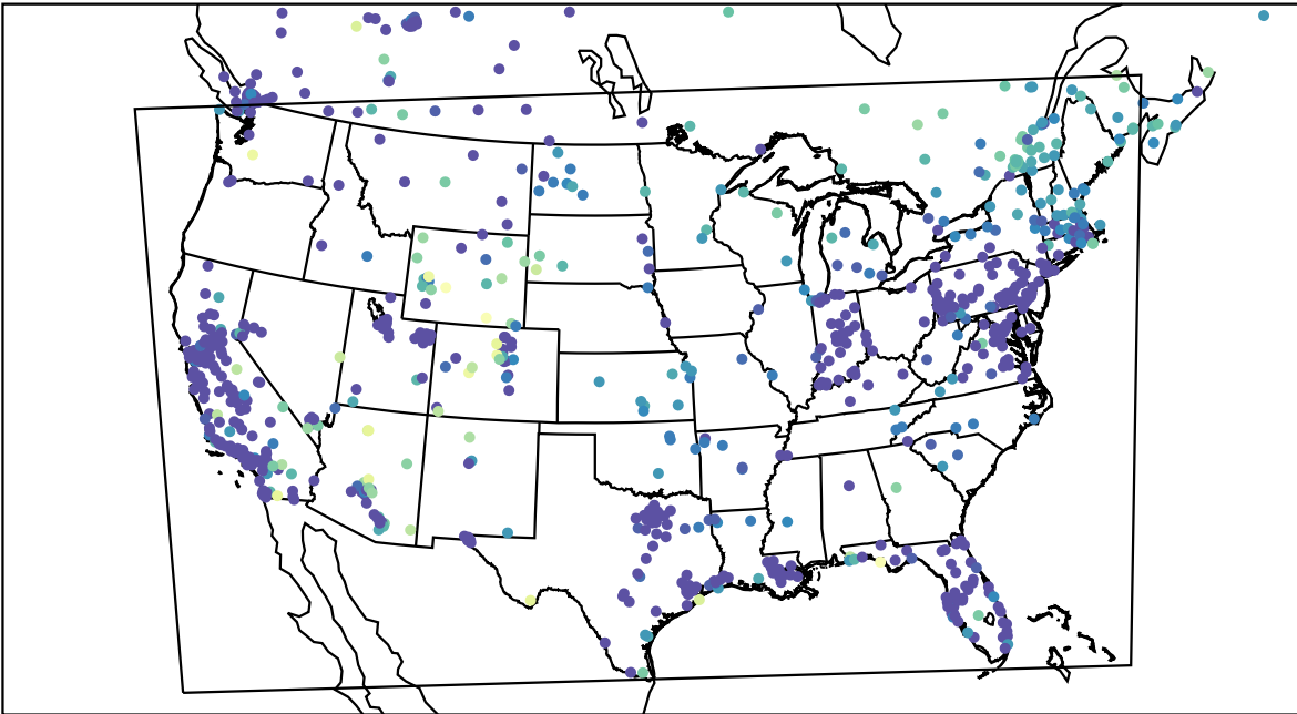
AirNOW (2024-01-01_08:00:00)
