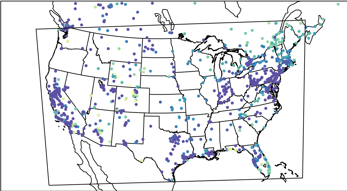
AirNOW (2024-01-01_14:00:00)
