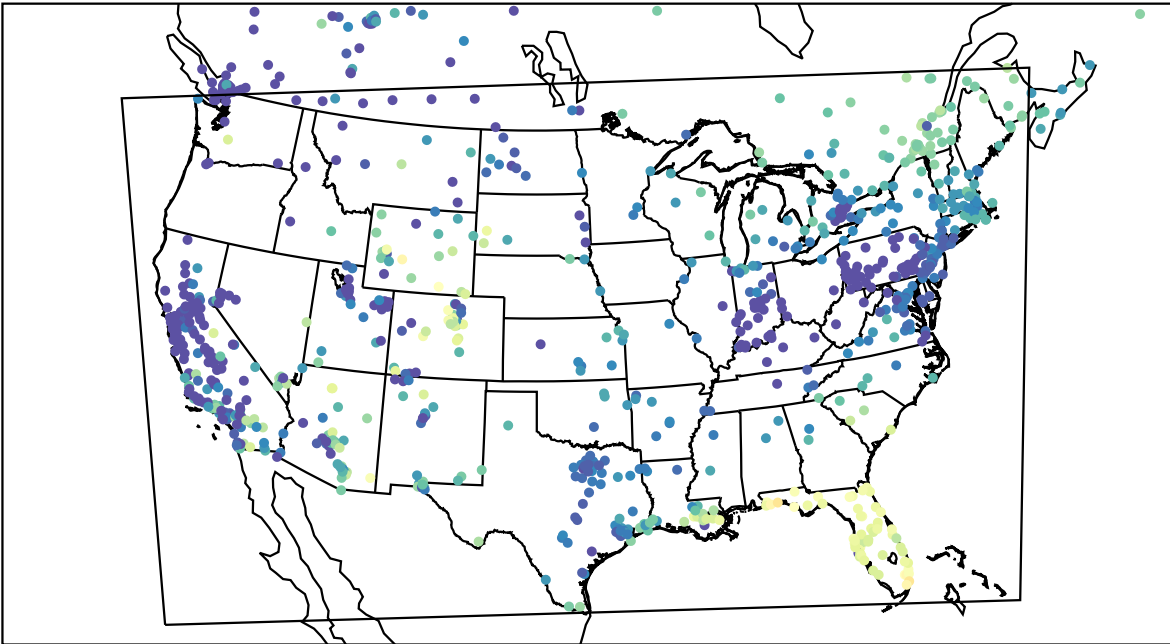
AirNOW (2024-01-01_17:00:00)
