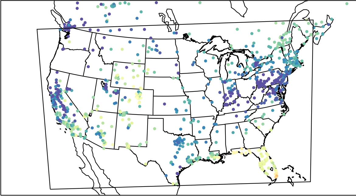
AirNOW (2024-01-01_19:00:00)
