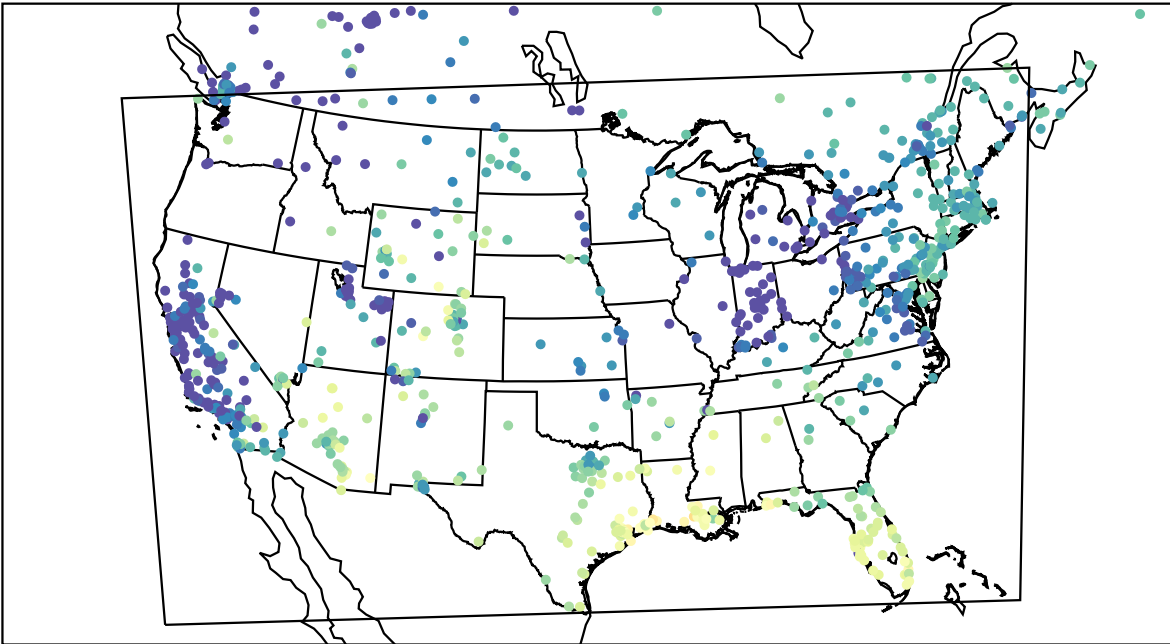
AirNOW (2023-12-31_18:00:00)
