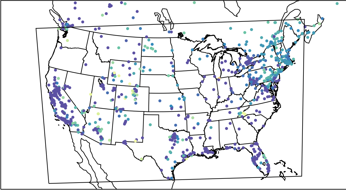
AirNOW (2023-12-31_10:00:00)
