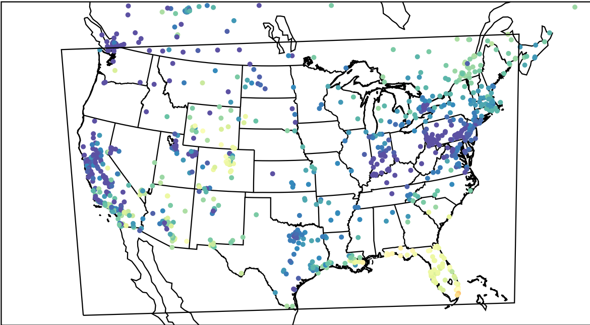
AirNOW (2024-01-01_18:00:00)
