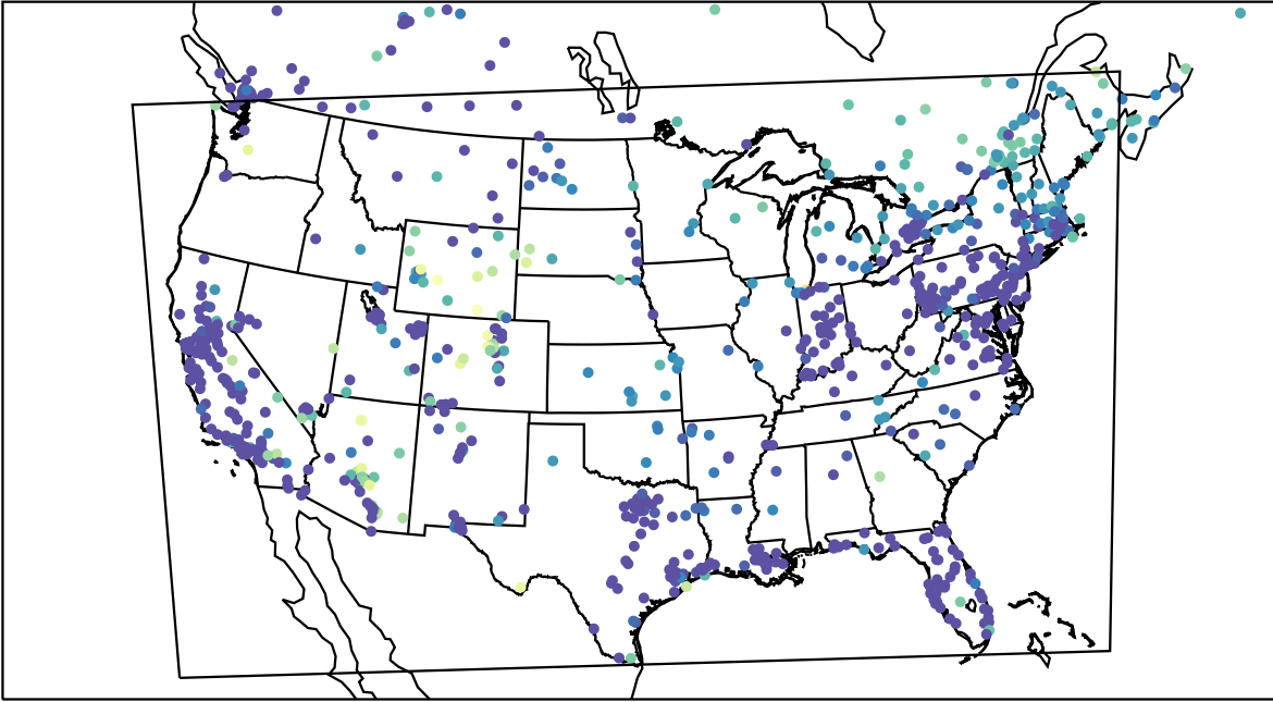
AirNOW (2024-01-01_10:00:00)
