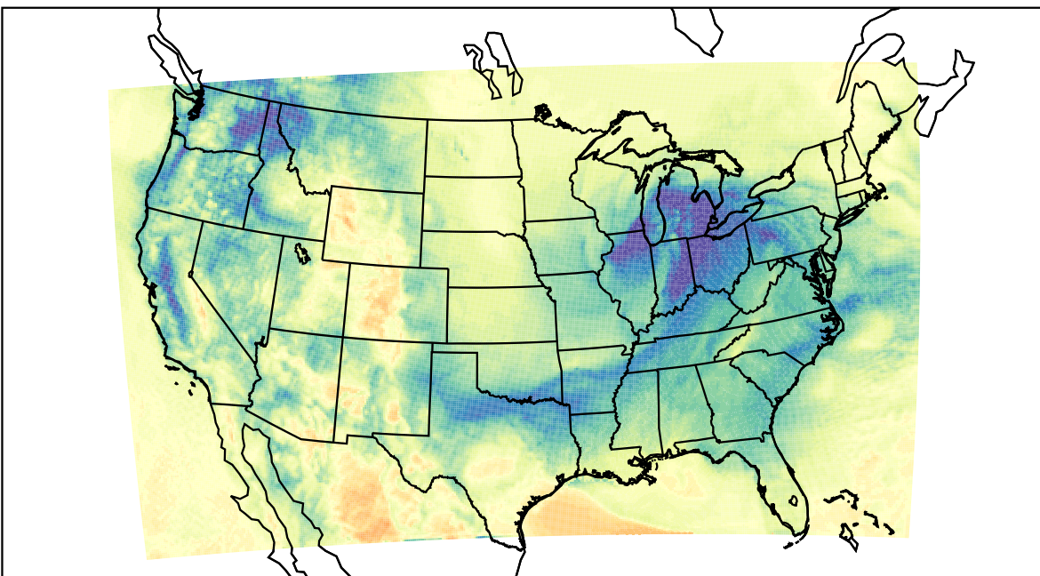
WRF (2023-12-31_18:00:00)
