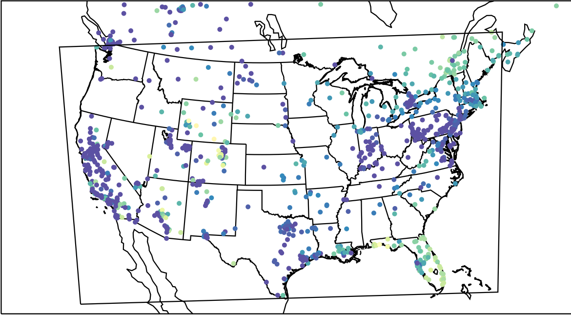
AirNOW (2024-01-01_15:00:00)
