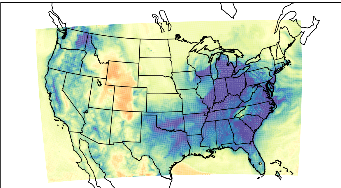
WRF (2023-12-31_13:00:00)
