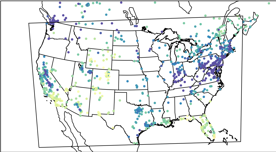
AirNOW (2024-01-01_22:00:00)
