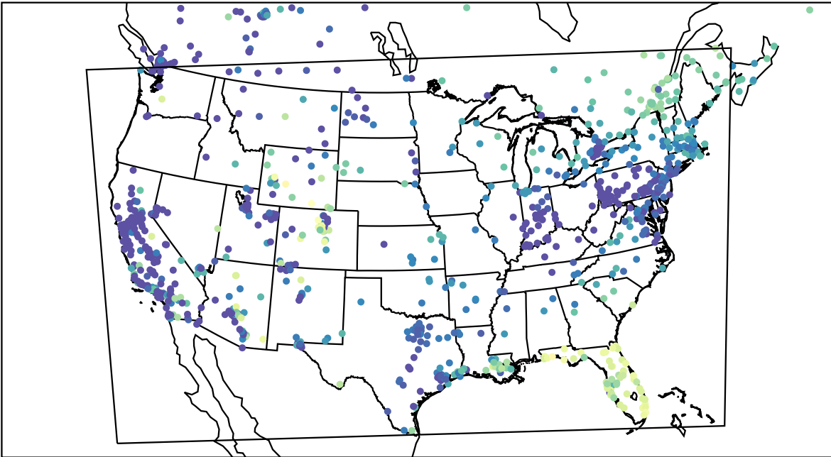
AirNOW (2024-01-01_16:00:00)
