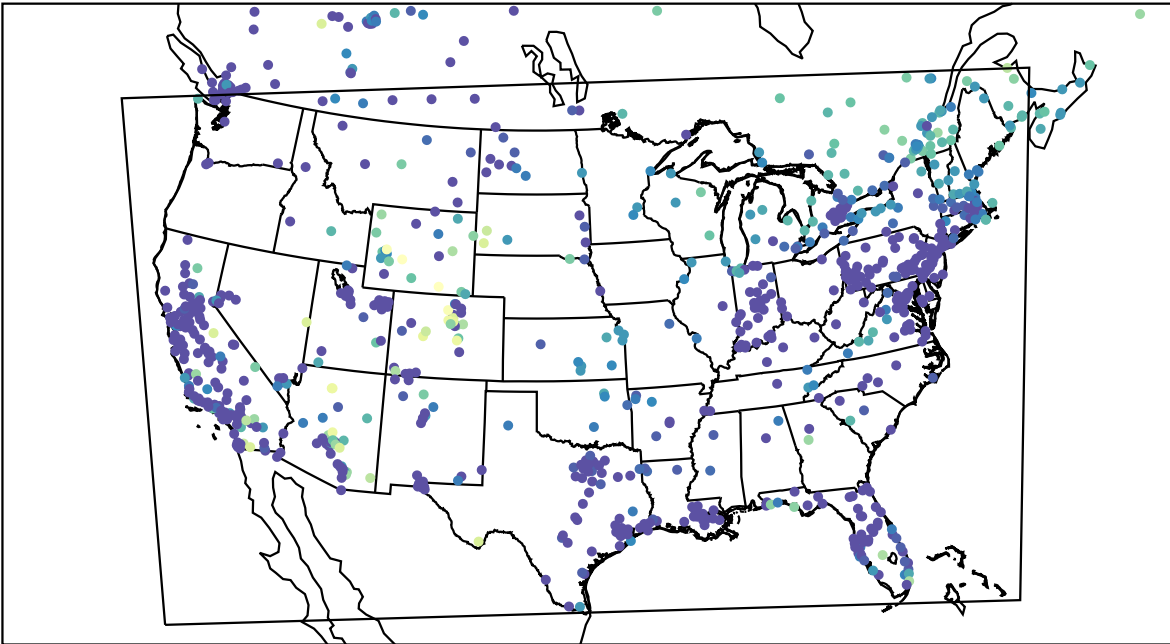
AirNOW (2024-01-01_13:00:00)
