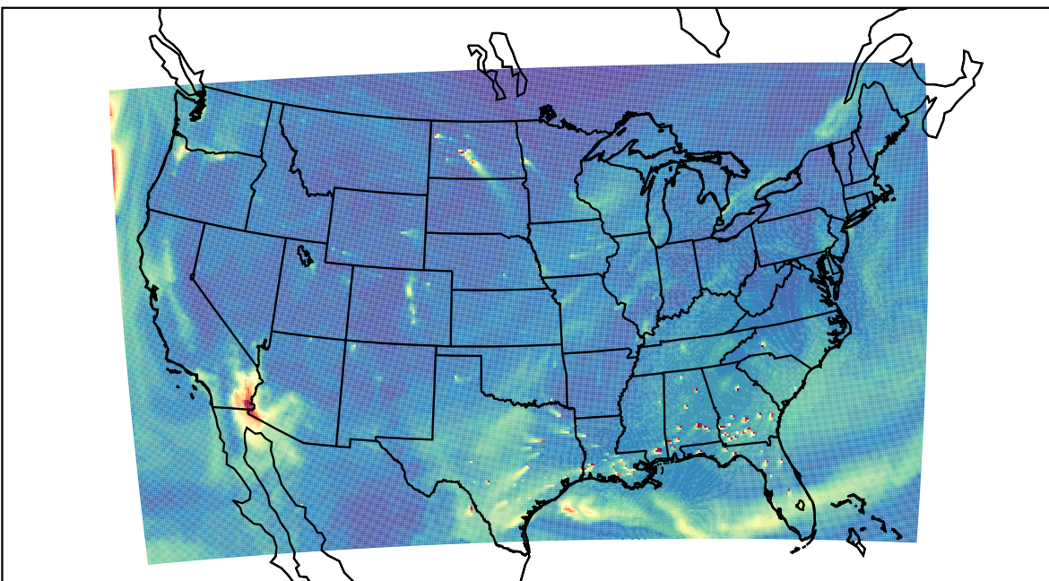
WRF 2024-01-02_18:00:00
