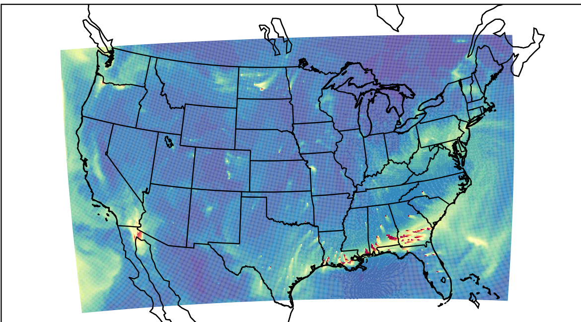
WRF 2024-01-01_20:00:00
