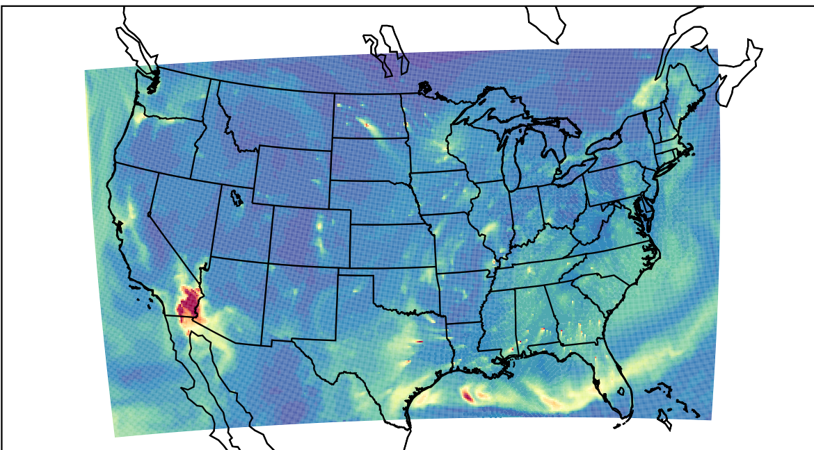
WRF 2024-01-02_13:00:00
