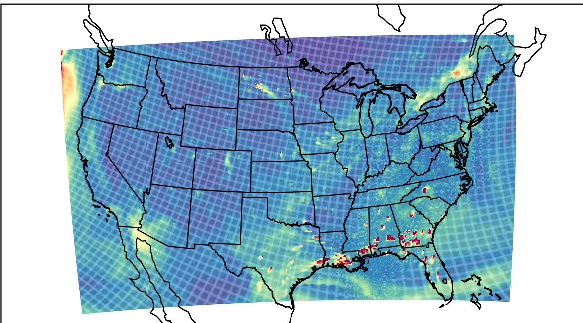
WRF 2024-01-02_23:00:00
