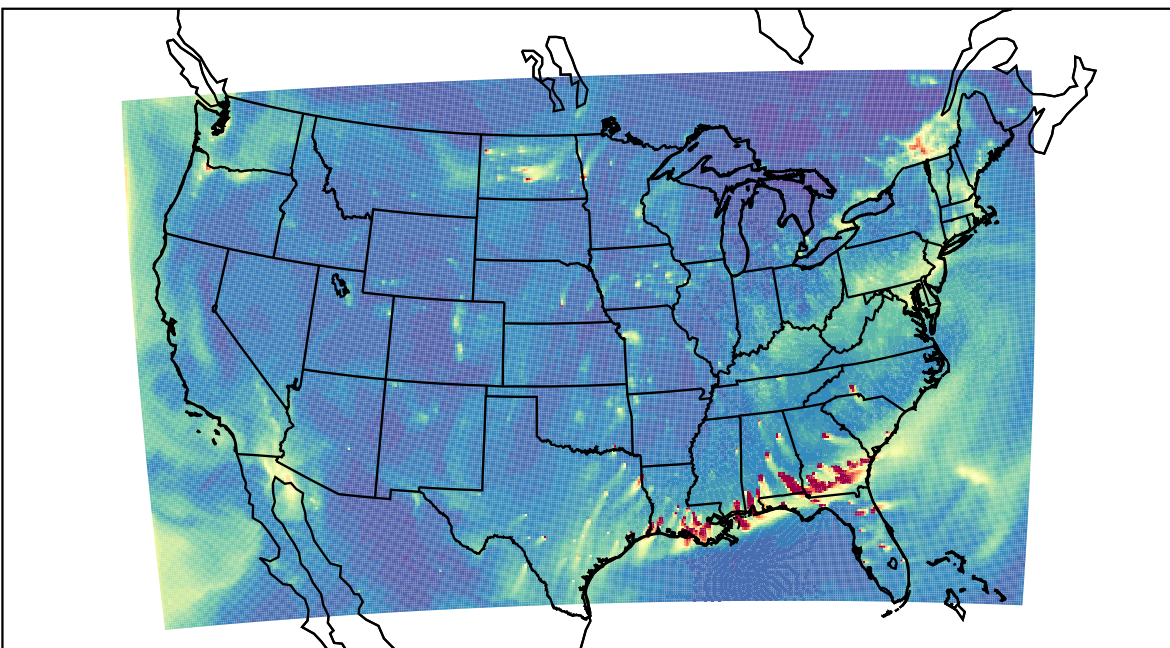
WRF 2024-01-01_23:00:00
