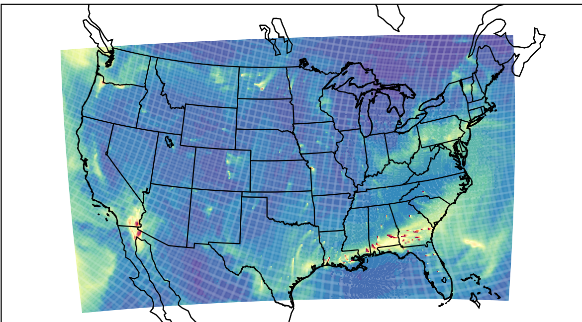
WRF 2024-01-01_18:00:00
