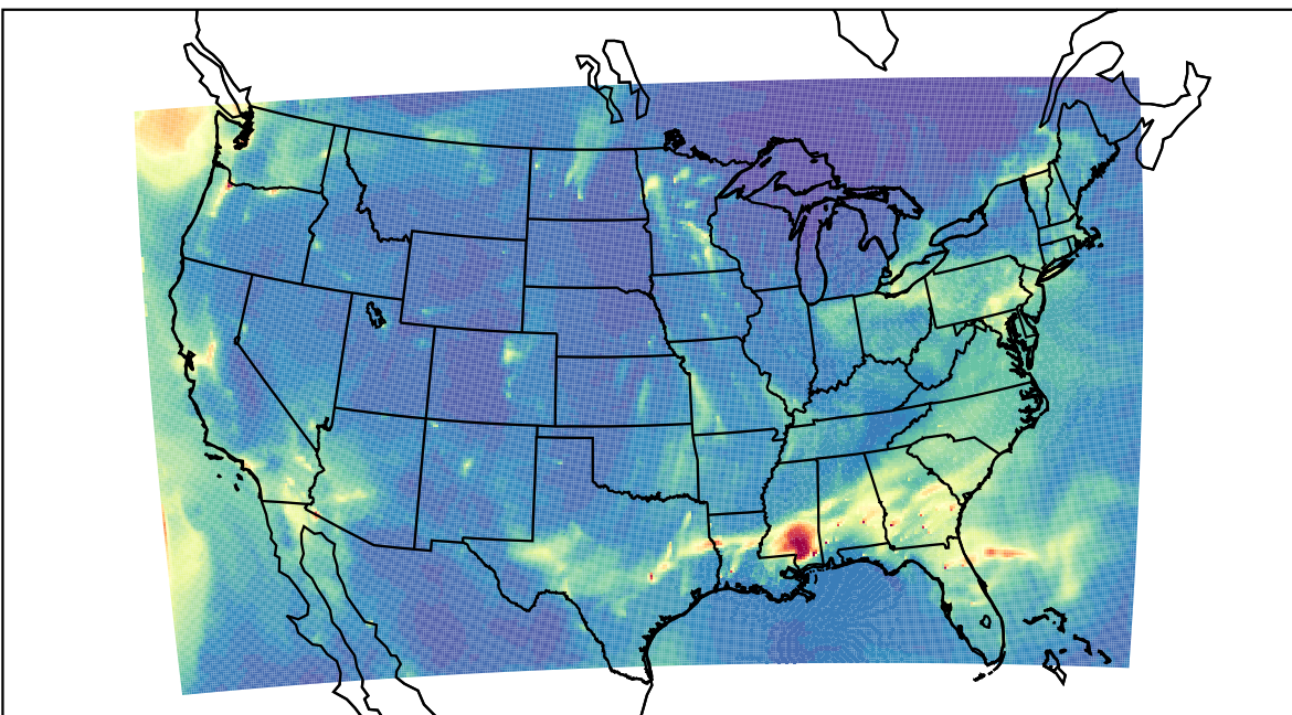
WRF 2024-01-01_09:00:00
