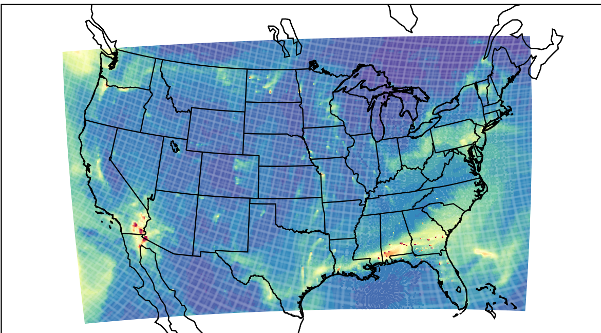
WRF 2024-01-01_16:00:00
