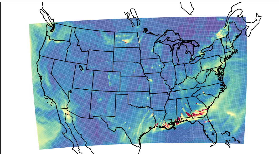
WRF 2024-01-01_22:00:00
