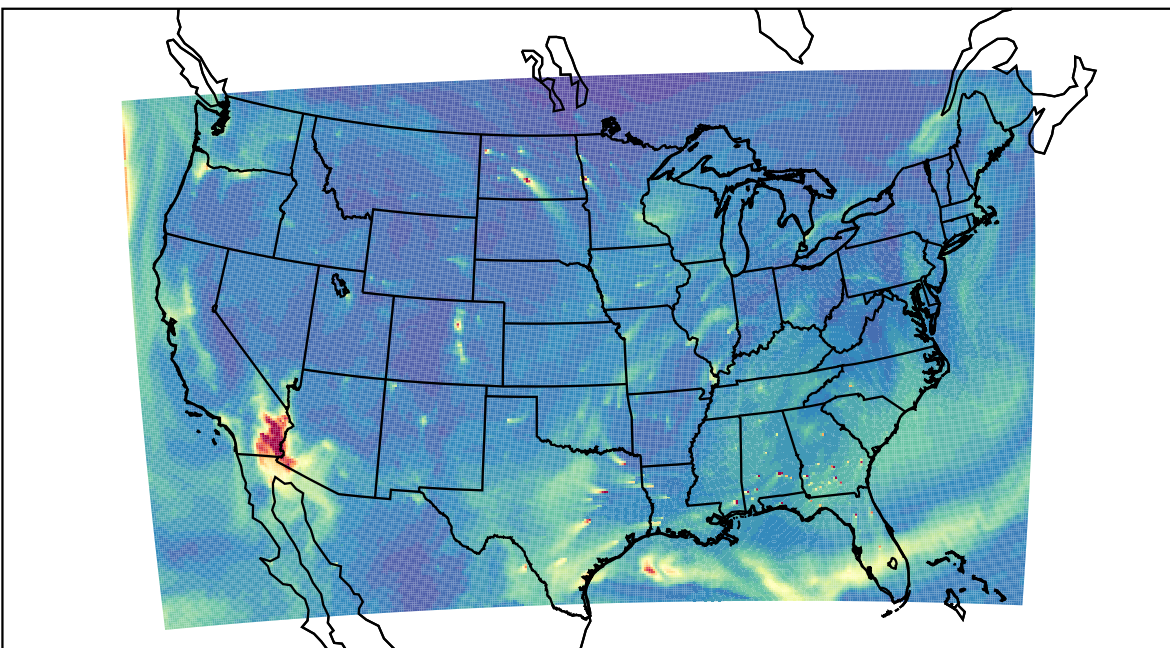
WRF 2024-01-02_16:00:00
