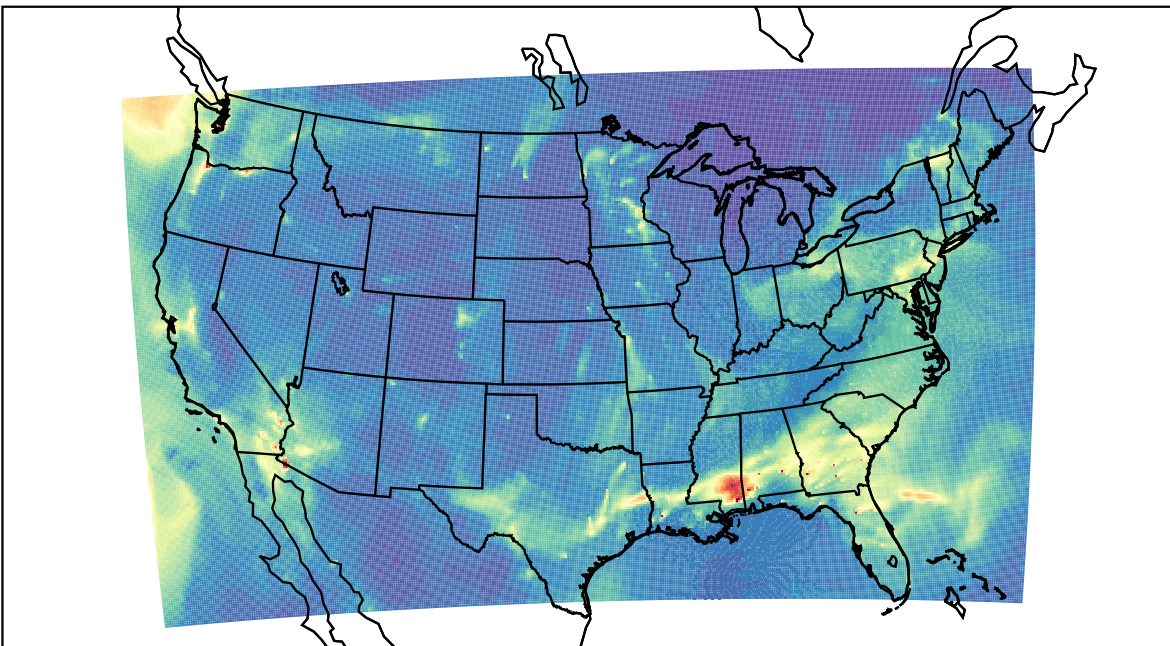
WRF 2024-01-01_11:00:00
