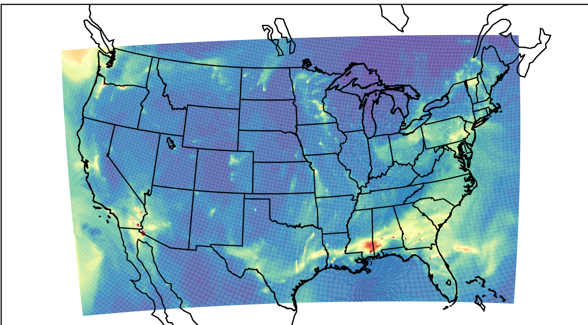
WRF 2024-01-01_12:00:00
