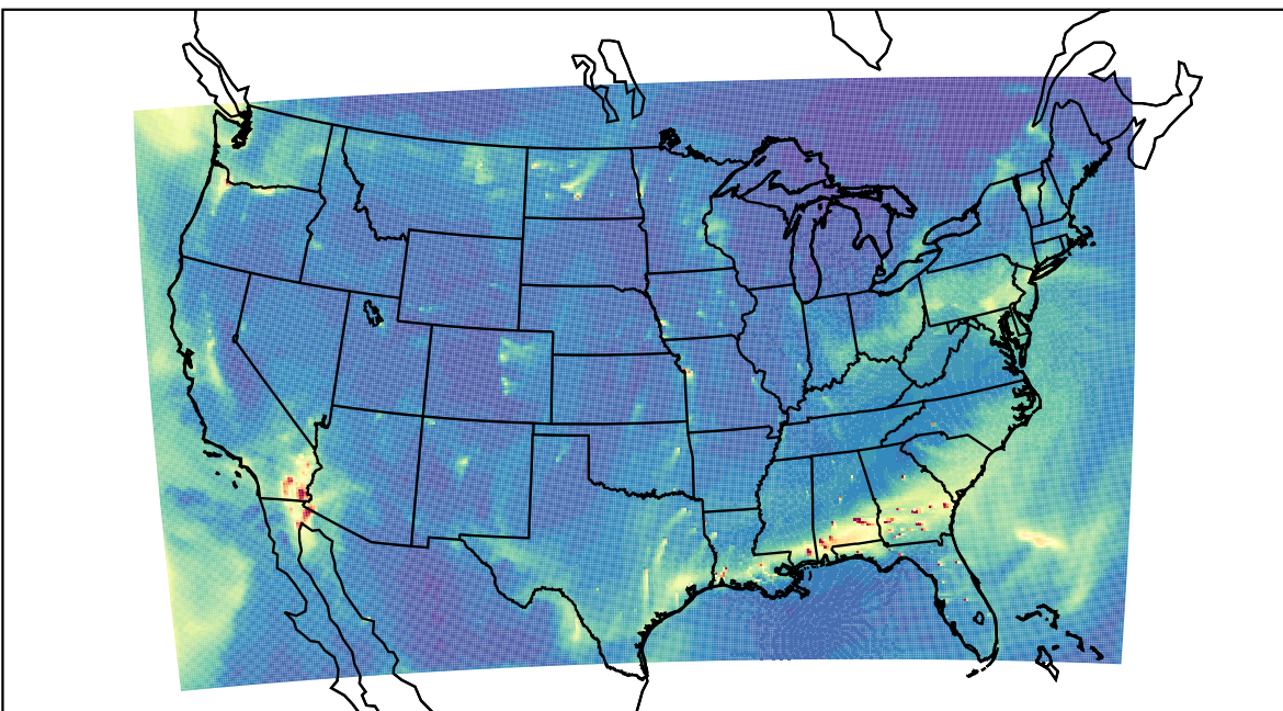
WRF 2024-01-01_17:00:00
