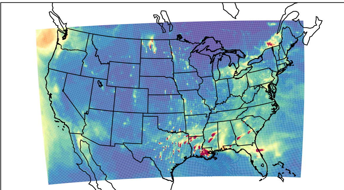
WRF 2024-01-01_00:00:00
