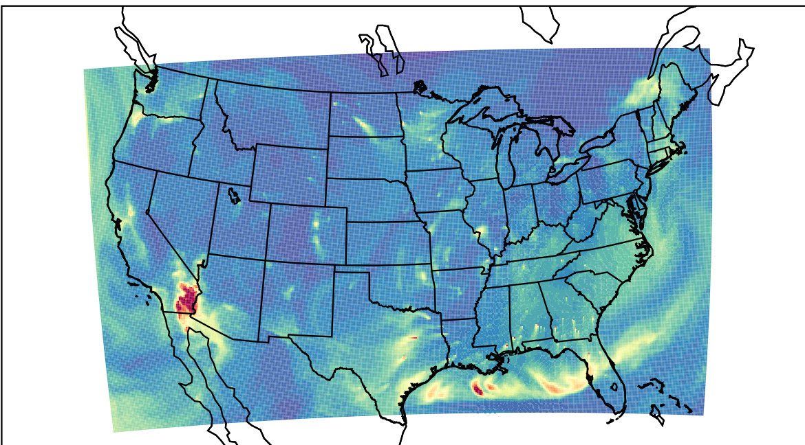
WRF 2024-01-02_10:00:00
