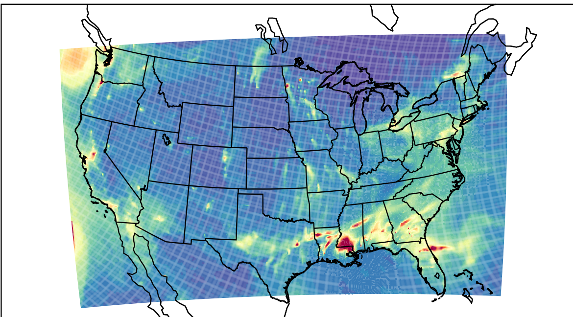
WRF 2024-01-01_06:00:00
