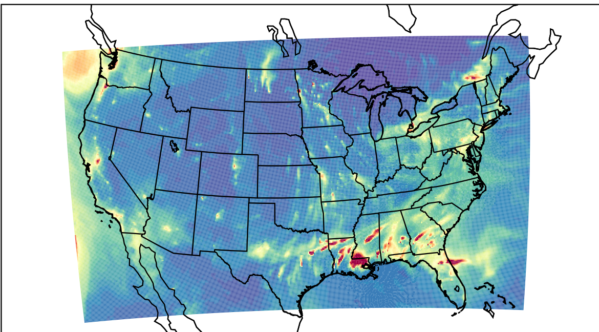
WRF 2024-01-01_04:00:00
