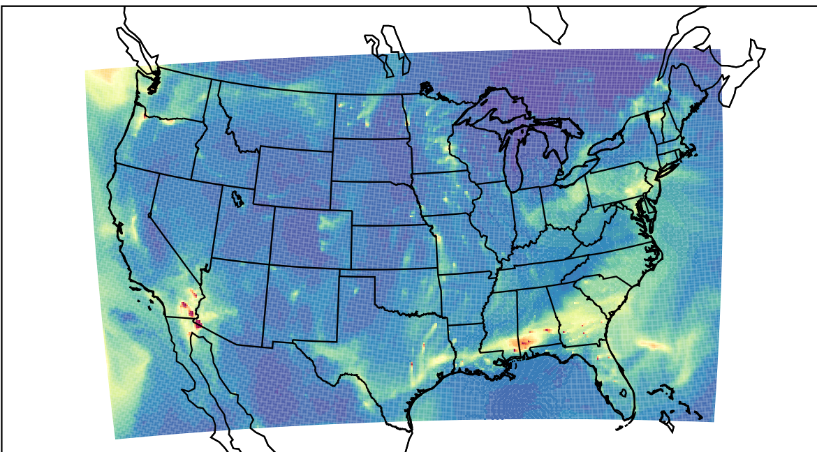
WRF 2024-01-01_14:00:00
