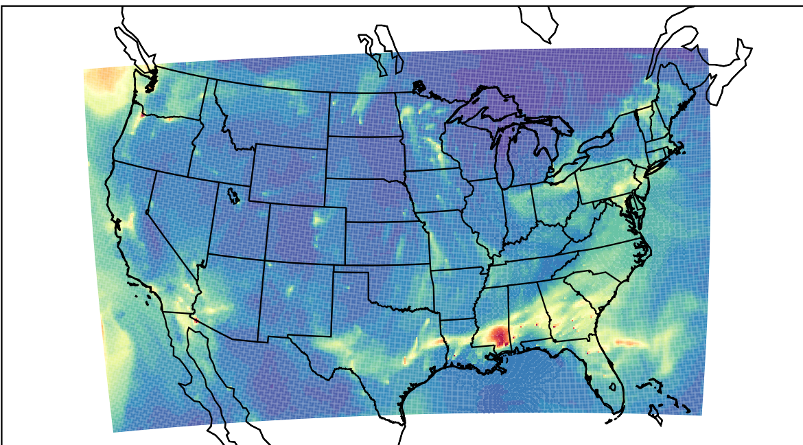
WRF 2024-01-01_10:00:00
