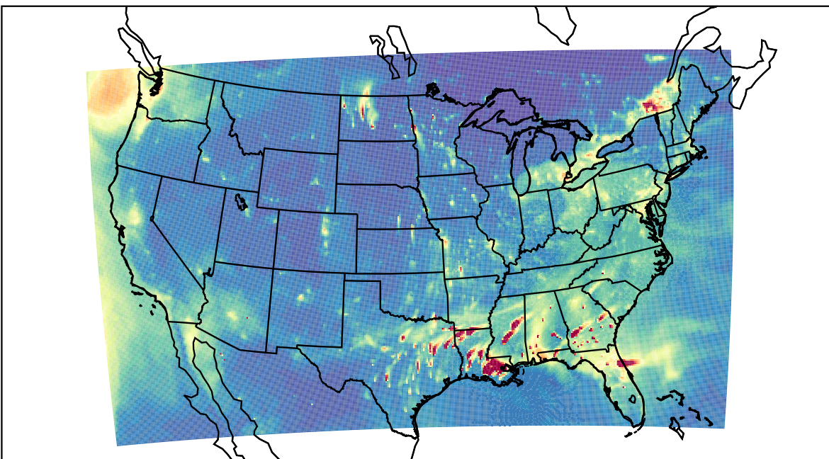
WRF 2024-01-01_01:00:00
