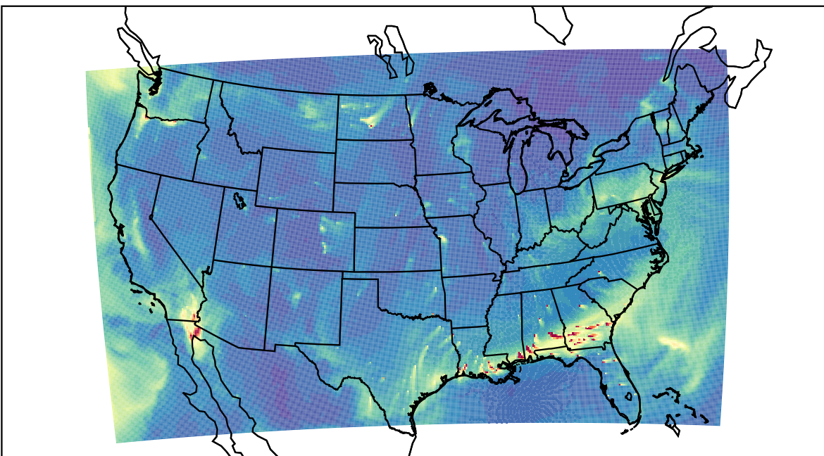
WRF 2024-01-01_19:00:00
