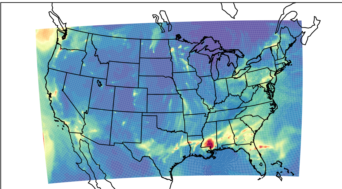
WRF 2024-01-01_08:00:00
