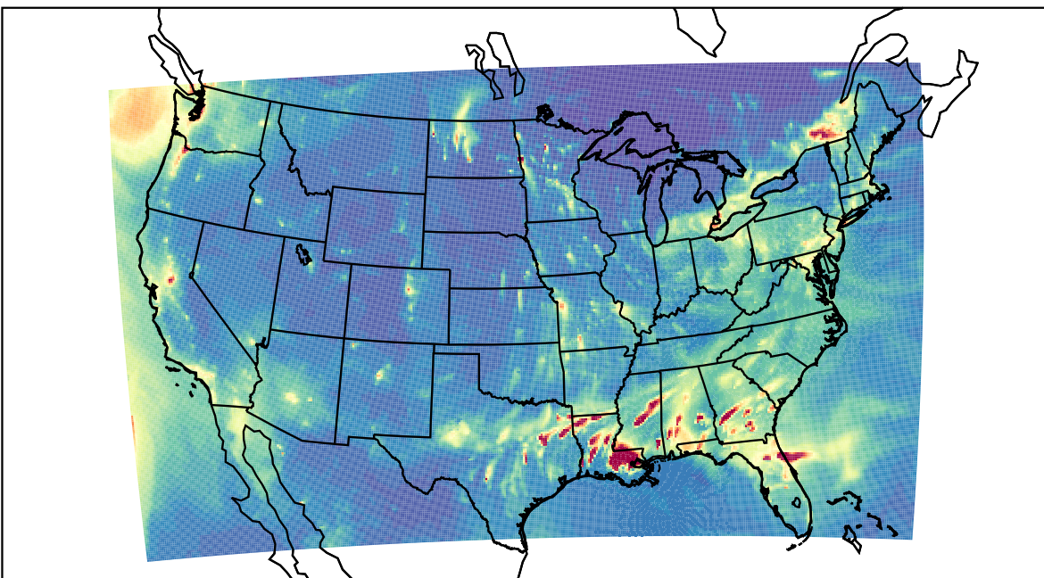
WRF 2024-01-01_03:00:00
