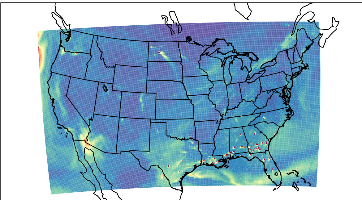
WRF 2024-01-02_20:00:00
