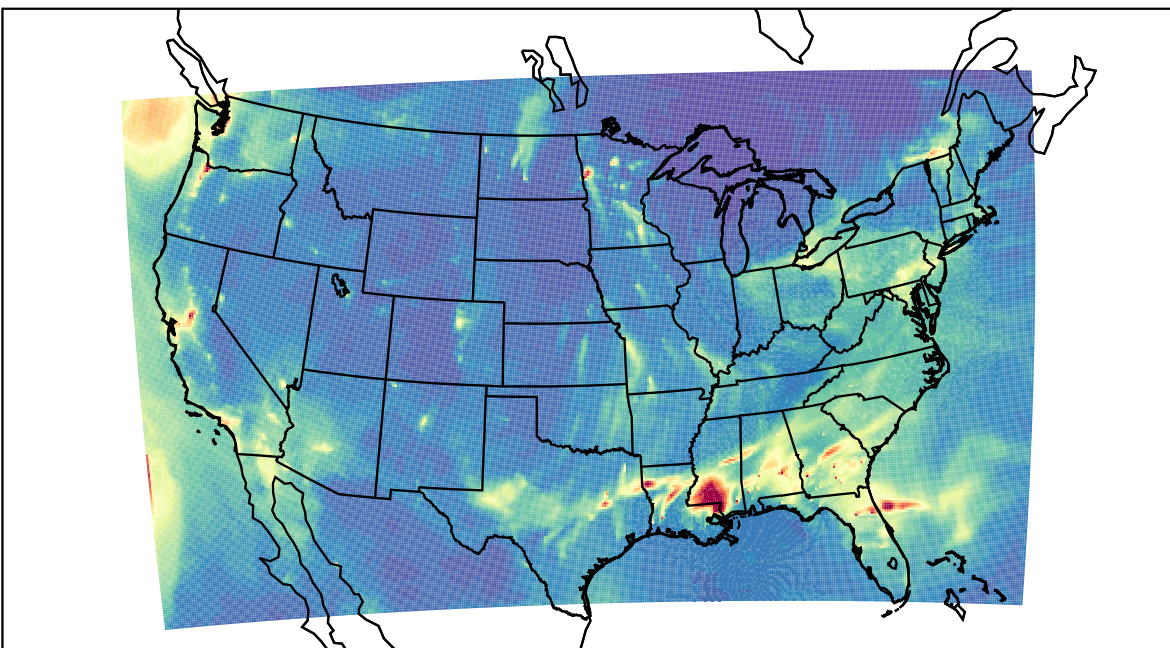
WRF 2024-01-01_07:00:00
