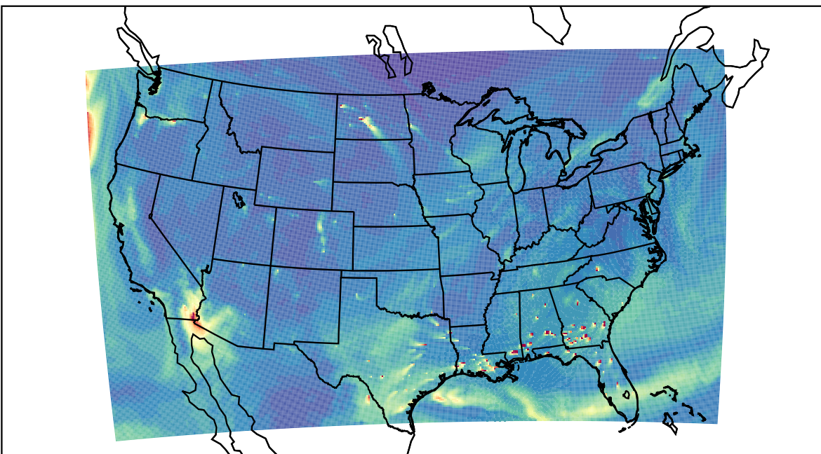
WRF 2024-01-02_19:00:00
