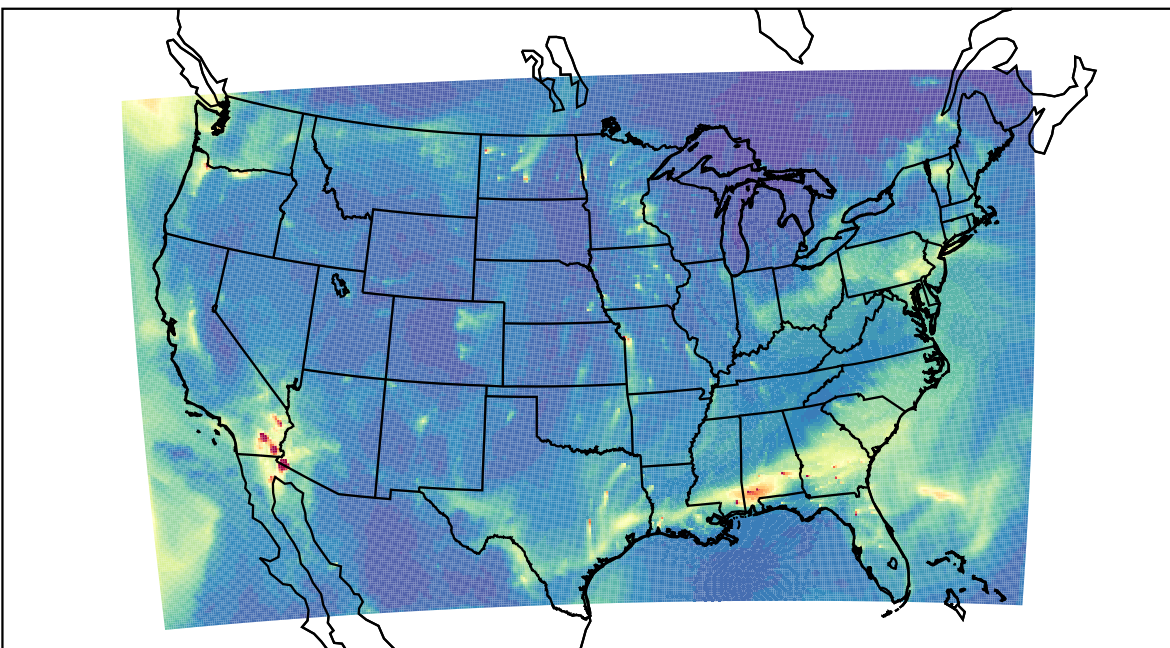
WRF 2024-01-01_15:00:00
