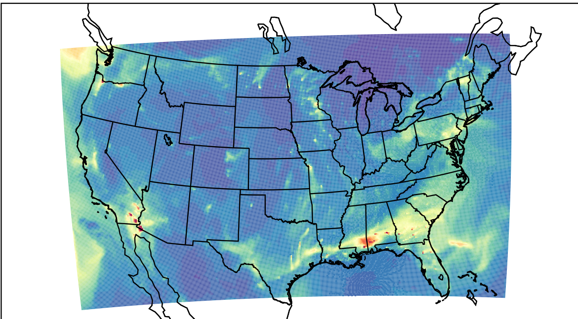
WRF 2024-01-01_13:00:00
