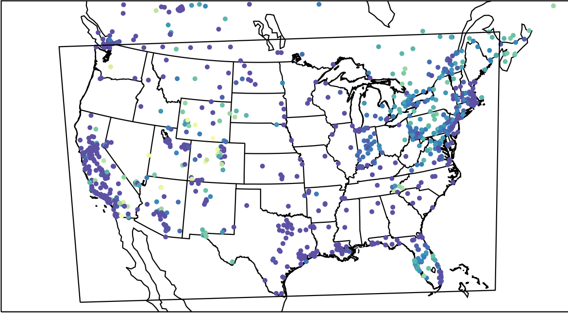
AirNOW (2024-01-02_13:00:00)
