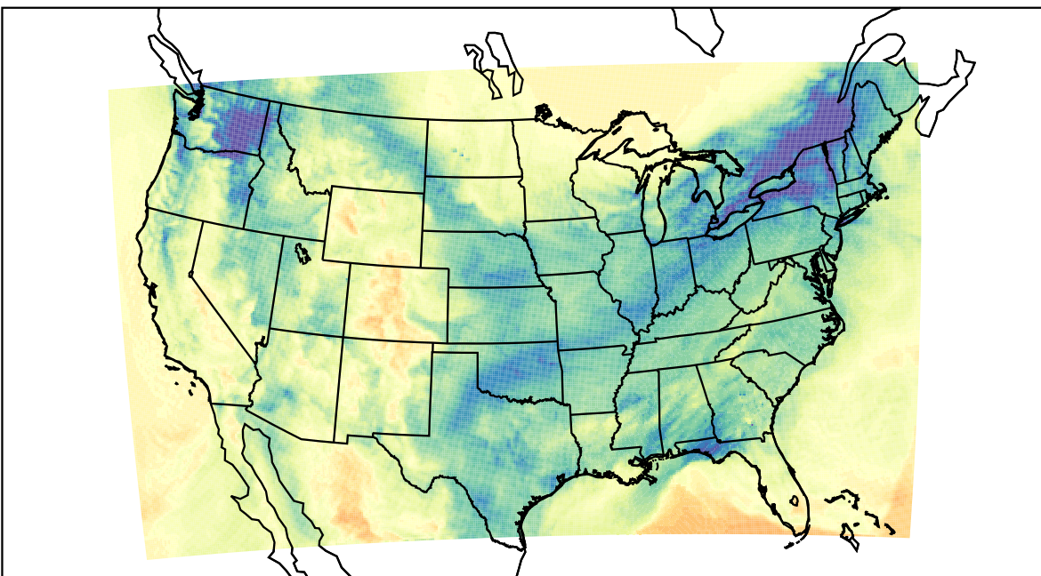
WRF (2024-01-03_20:00:00)
