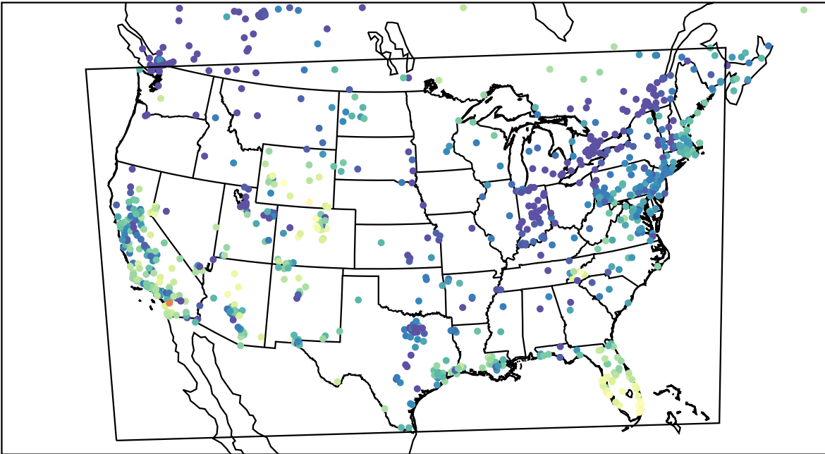
AirNOW (2024-01-03_18:00:00)
