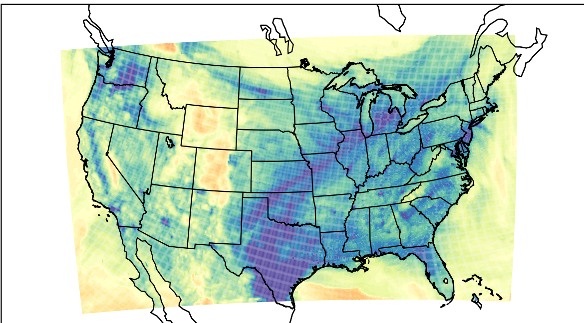
WRF (2024-01-03_04:00:00)
