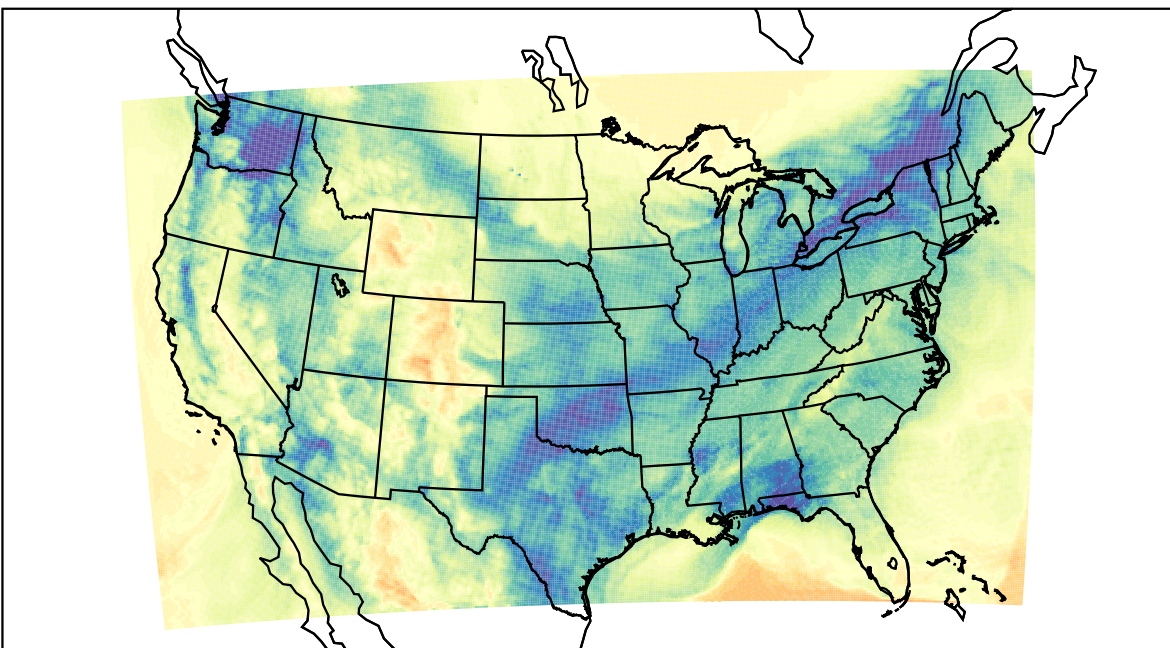
WRF (2024-01-03_18:00:00)
