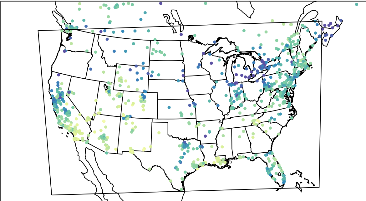
AirNOW (2024-01-11_18:00:00)
