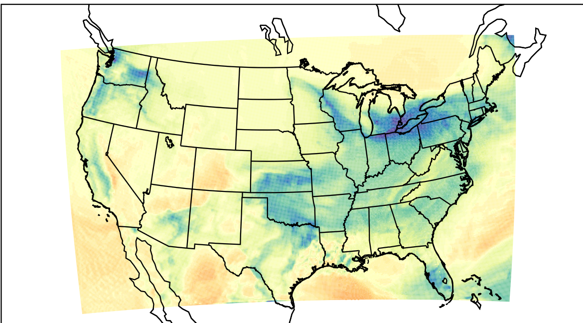
WRF (2024-01-11_18:00:00)
