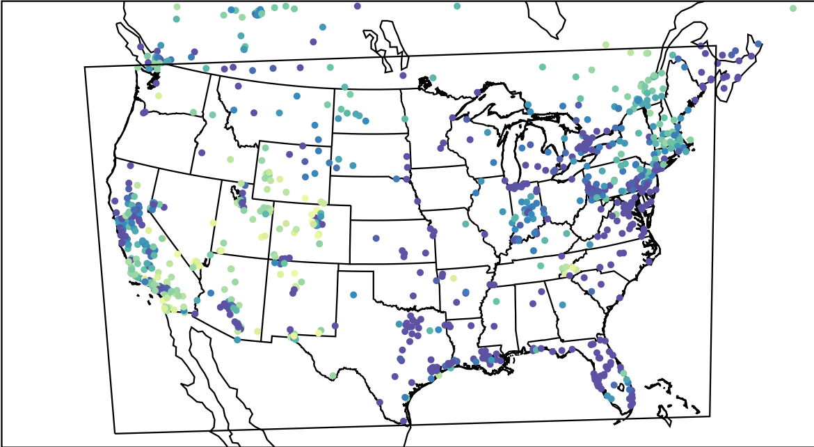
AirNOW (2024-01-11_13:00:00)
