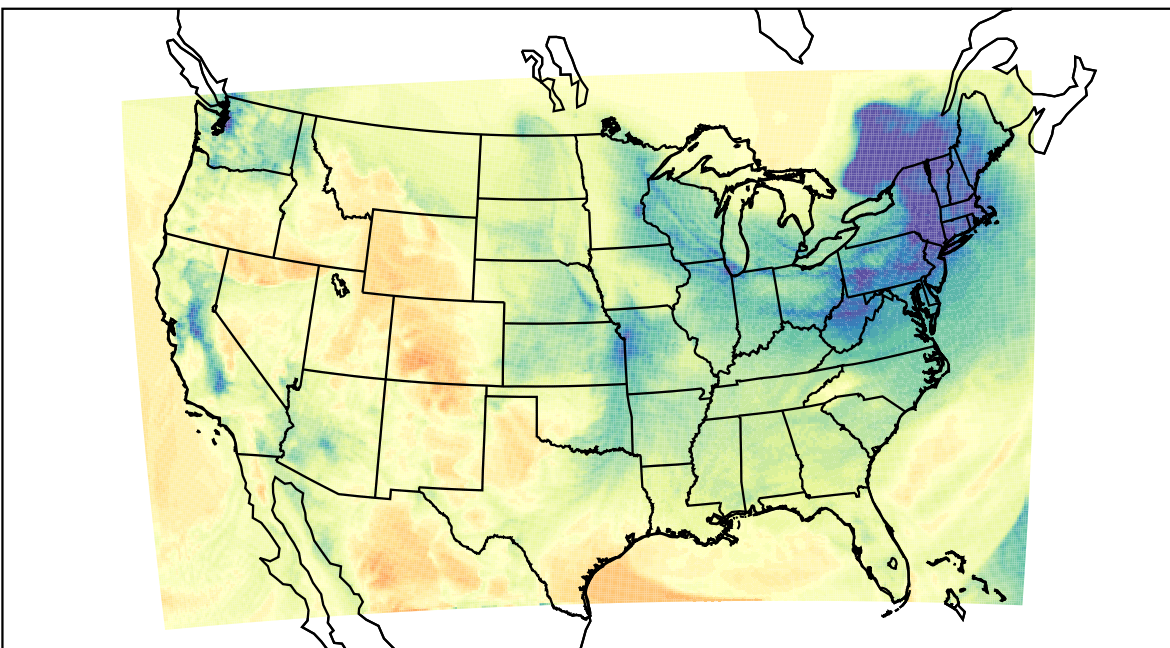
WRF (2024-01-10_20:00:00)
