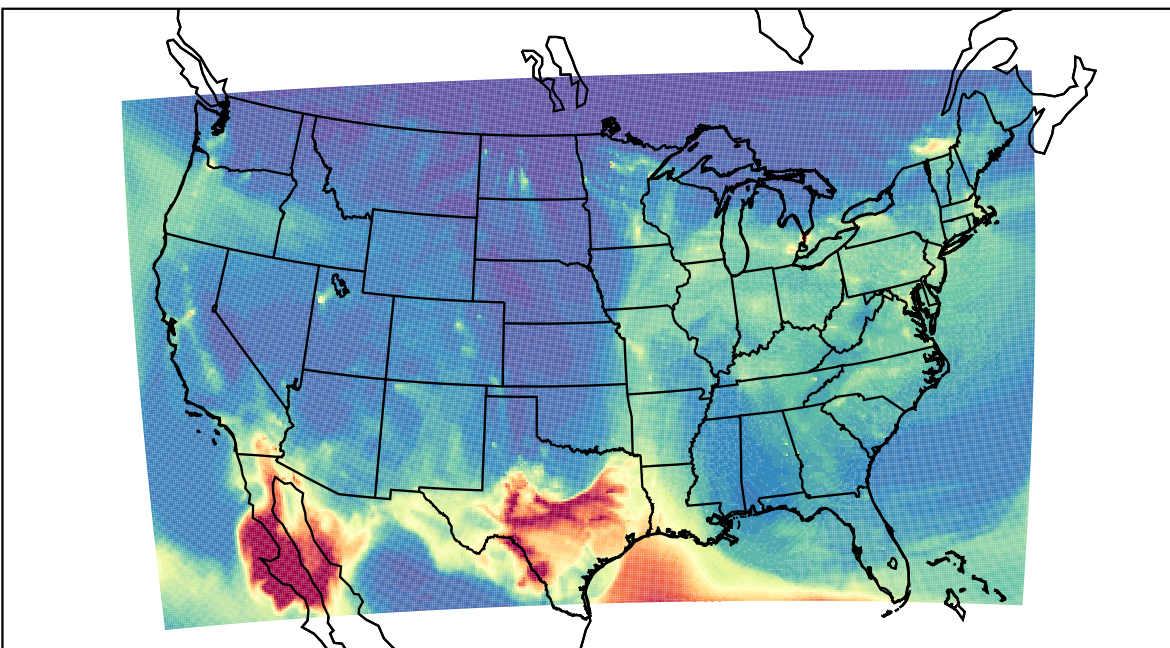
WRF 2024-01-12_10:00:00
