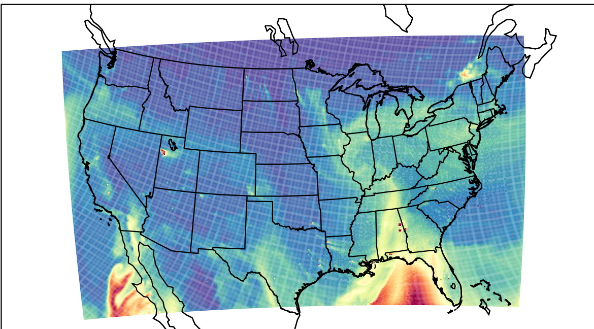
WRF 2024-01-12_20:00:00
