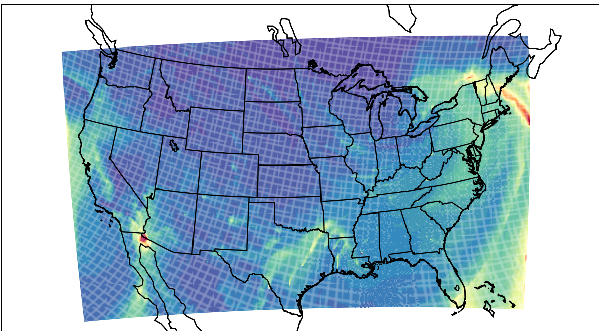
WRF 2024-01-13_18:00:00
